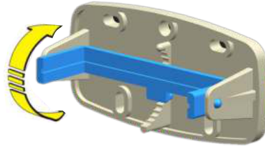
Şekil 2 : Algılama Açısının Ayarlanması Figure 2: Calibration Angle Adjustment
