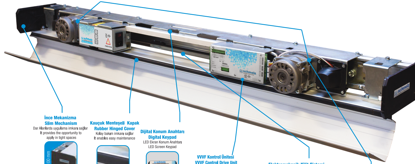
Elektromekanik Kilit Sistemi Electromechanic Lock System Step motorlu kilit sayesinde sürekli çalışma sağlar Step motor lock ensures continuous operation
