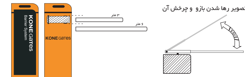
۴ مدل گارد آنتی کرش (ضد لح) با بازوی آلومینیوم رها شونده ۳ تا ۶ متر
